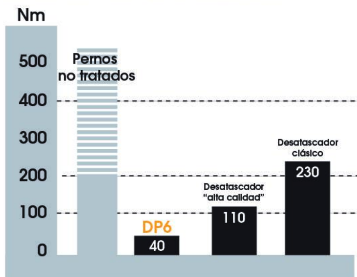
TEST MIL A 907 - E/D: par de aflojamiento
