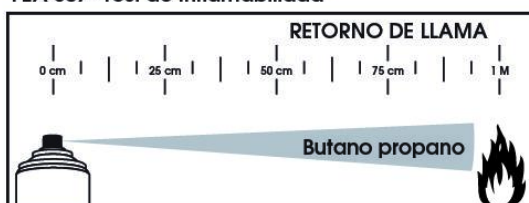
FEA 607- Test de inflamabilidad
