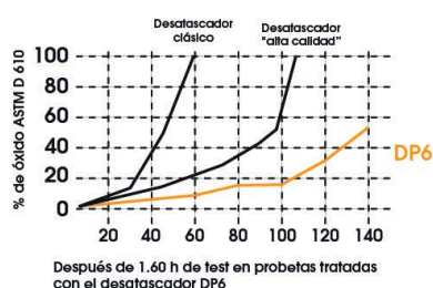
Habitación húmeda - norma ASTM D 2247
