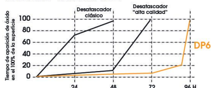
Niebla salina - norma NFX 41002
